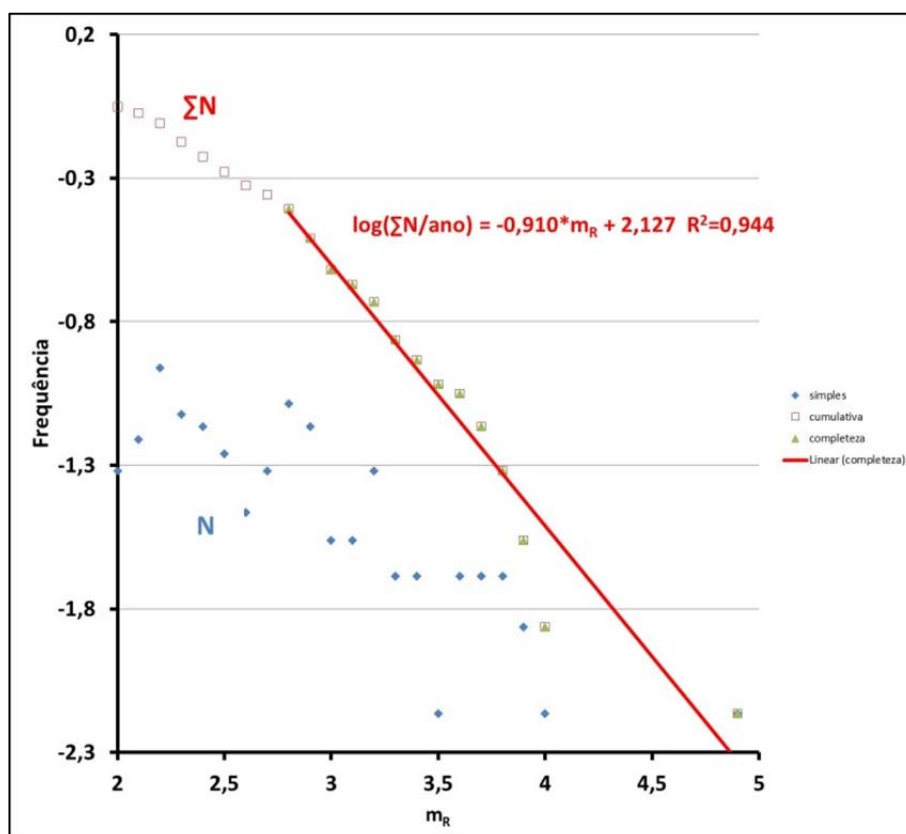
Figura 3.6 – Relação Frequência – Magnitude de GUTENBERG-RICHTER.
