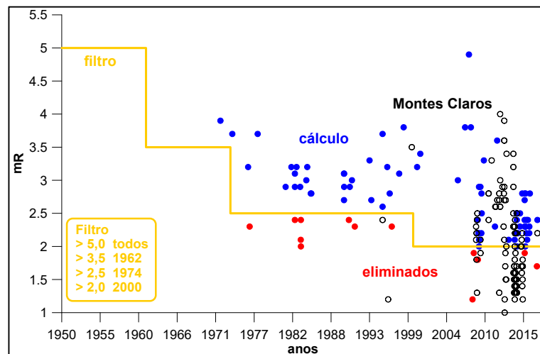
Figura 3.5 – Distribuição temporal dos sismos de Montes Claros.
