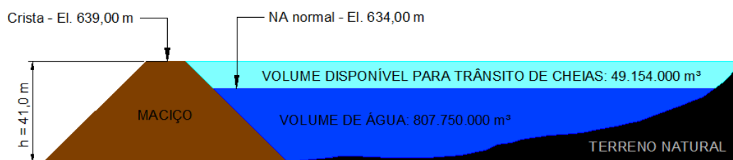
FIGURA 6 – RESERVATÓRIO DA BARRAGEM DO RIO VACARIA.
