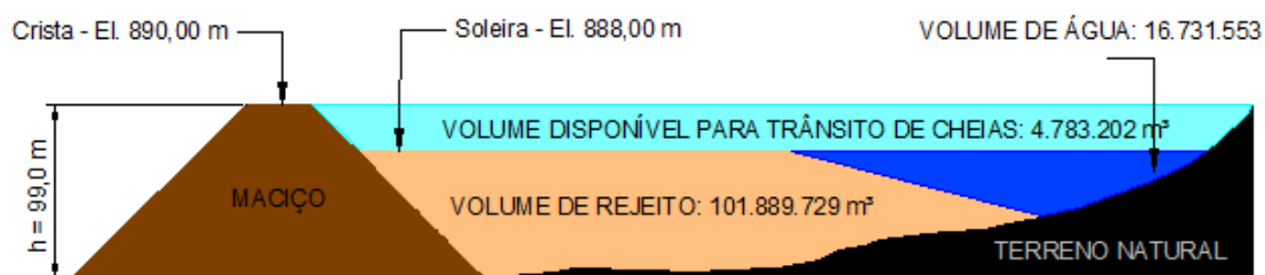
FIGURA 6 – RESERVATÓRIO DA BARRAGEM 2.
