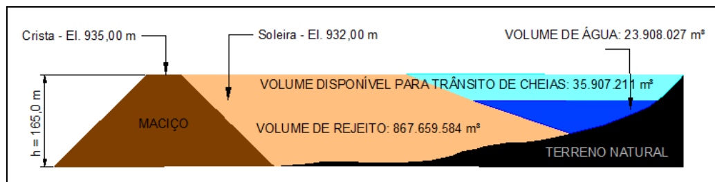
FIGURA 6 – RESERVATÓRIO DA BARRAGEM 1.
