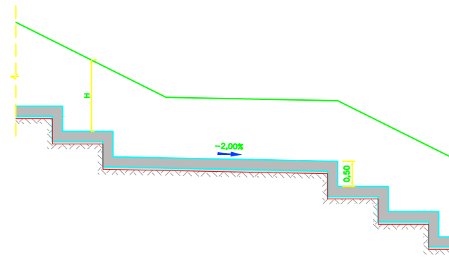
PERFIL TÍPICO – CANAL PERIFÉRICO SEM ESCALA
