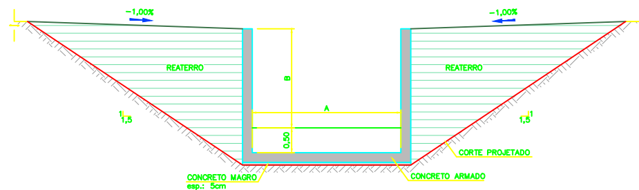
SEÇÃO TÍPICA – CANAL PERIFÉRICO EM DEGRAU SEM ESCALA
