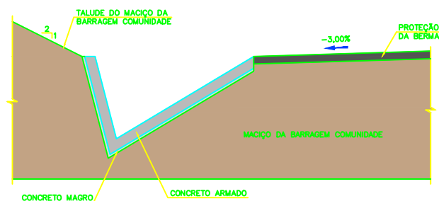
DETALHE TÍPICO – CANALETA DE BERMA TRIANGULAR SEM ESCALA
