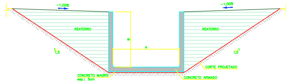
SEÇÃO TÍPICA – CANAL PERIFÉRICO SEM ESCALA
