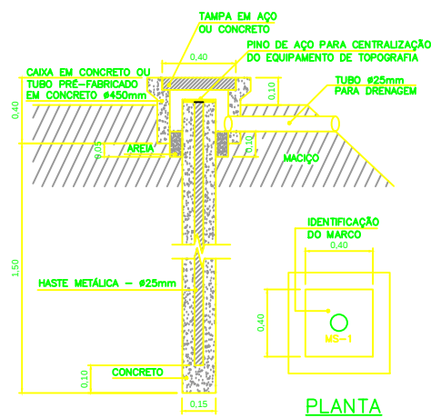
MARCO TOPOGRÁFICO (MS) SEM ESCALA
