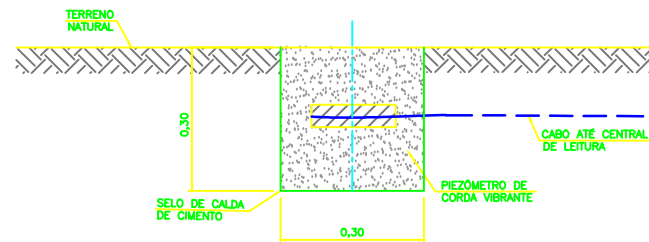
DETALHE PIEZÔMETRO ELETRÔNICO DE CORDA VIBRANTE SEM ESCALA
