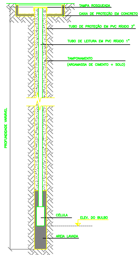
PIEZÔMETRO CASAGRANDE (PZC) SEM ESCALA
