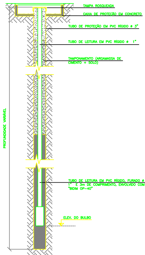
MEDIDOR DE NÍVEL D'ÁGUA (MNA) SEM ESCALA
